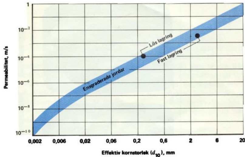
Figur 7.2 – 7 Överslagsvärden på permeabiliteten hos kornfraktioner och ensgraderade jordar
