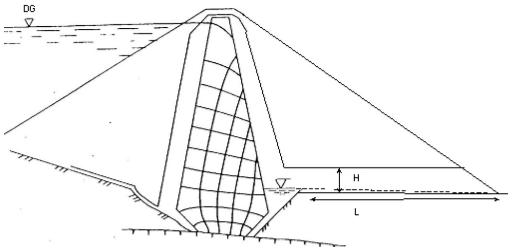
Figur 7.2 – 2 Dimensionering av läckage i dammkroppen för normal genomläckning
