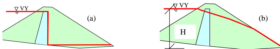
Figur 7.2 – 6 Normal tryckfördelning dammkroppen (a) och antagen tryckfördelning vid dimensionerande läckage (b)
