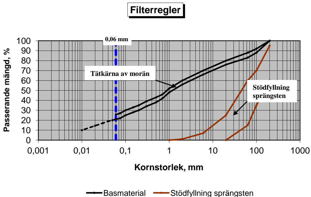
Figur 7.2 – 3 Envelopper för basmaterialets och stödfyllningens kornfördelning
