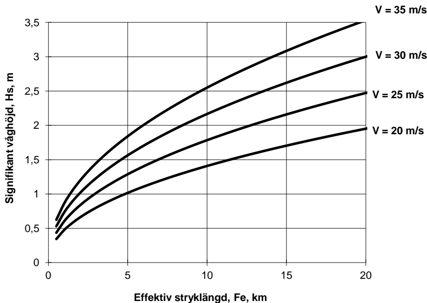
Figur 7.2 – 10 Signifikanta våghöjden som funktion av effektiva stryklängden
