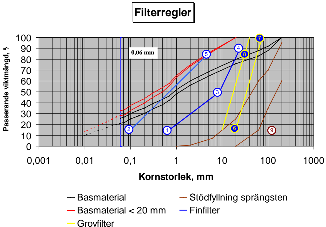
Figur 7.2 – 4 Exempel på utformning av ett finfilter och ett grovfiler vid ett givet basmaterial och en given stödfyllning.
