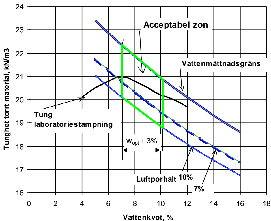
Figur 7.2 – 1 Acceptabel zon för moränens tunghet för torrt material, vattenkvot och luftporhalt vid packning (tunghet för kornen 26,5 \text{ kN/m}^3 )
