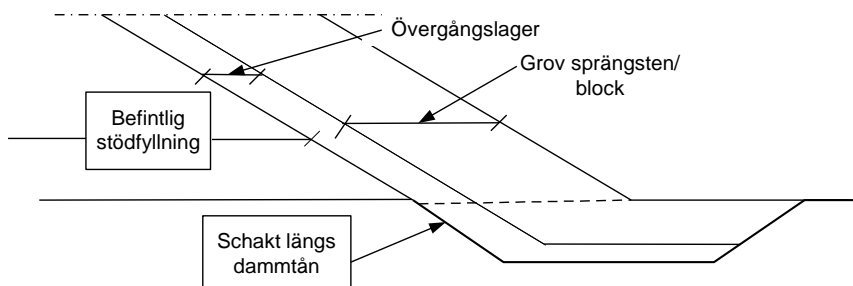
Figur 7.2 – 9 Utformning av skyddsvall där dammens stödfyllning är grundlagd på jord
