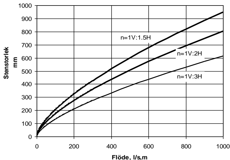
Figur 7.2 - 8 Erforderlig stenstorlek ur erosionssynpunkt i förhållande till utströmmande flödet
