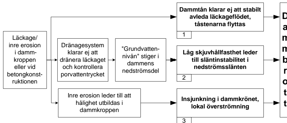
Figur 7.2- 5 Brottförlopp initierade av läckage/inre erosion i dammkroppen eller valvbildning längs betongkonstruktionen
