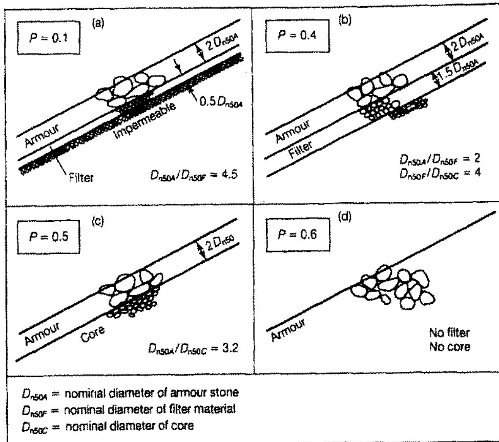
Figur 7.2-11 Riktlinjer för bestämning av permeabilitetsparametern, P, enligt van der Meer [3.2 – 56]. Observera att D_{n50} = 0,84 \cdot D_{50} samt att 'Core' i bild (c) avser stödfyllning.
