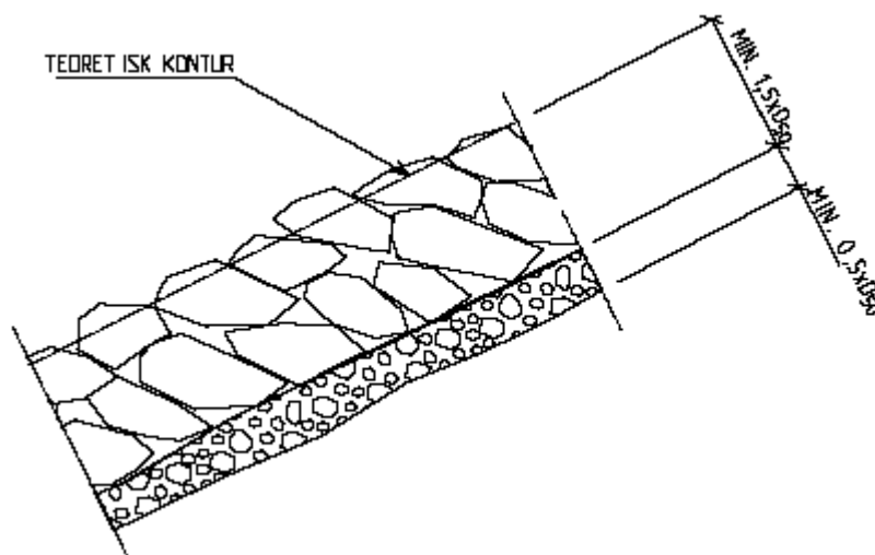
Figur 7.2-12 Utformning av erosionsskydd (princip).
