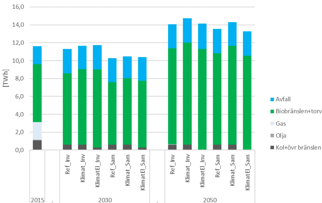
Figur 40. Elproduktionen från kraftvärmeverk i de svenska fjärrvärmenäten (dvs. ej industri).
