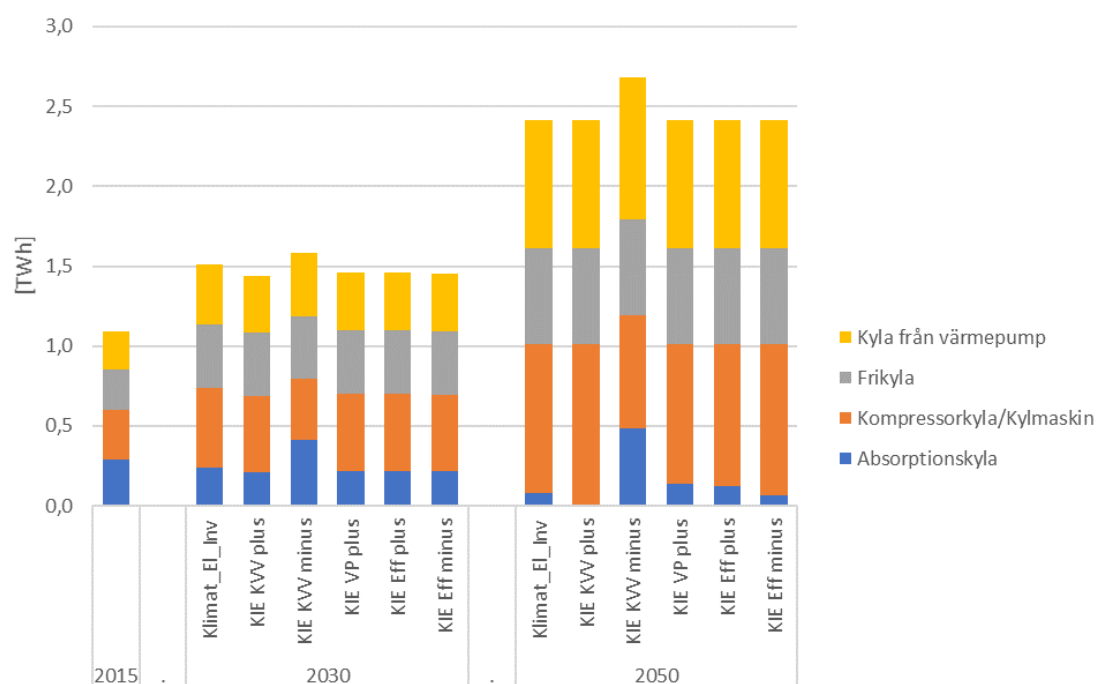
Figur 49. Fjärrkylproduktion i grundscenariot KlimatEL_Inv inklusive olika teknikscenarier.
