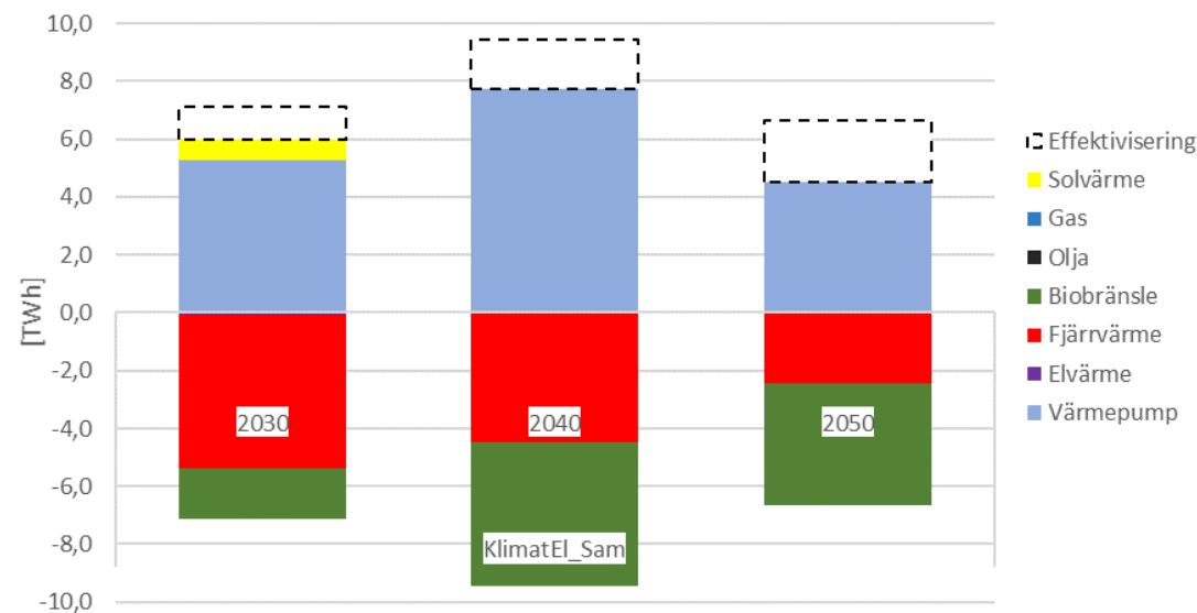
Figur 31. Nyttiggjord energi för uppvärmning i bostäder och lokaler, KlimatEI_Sam skillnad mot KlimatEI_Inv.
