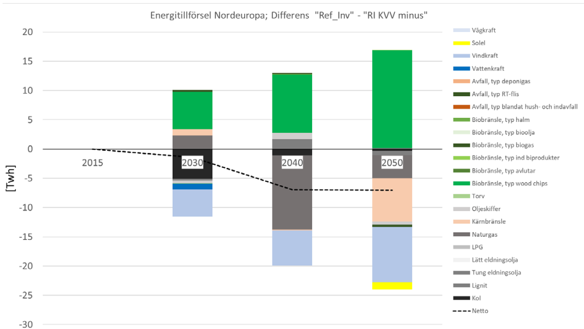
Figur 41. Skillnaden i primärenergitillförsel på Nordeuropainivå mellan ett fall där nyinvesteringar i svensk kraftvärme tillåts (Ref_Inv) och ett fall där sådana investeringar inte tillåts (RI KVV minus).
