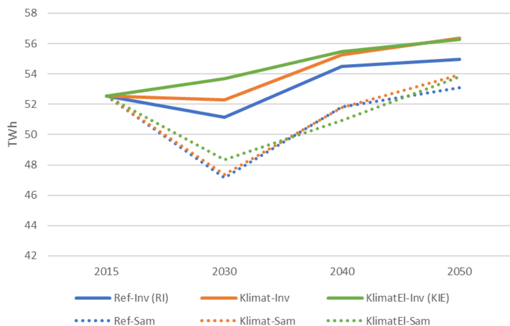
Figur 32. Potentialbedömning för fjärrvärmeleveranser.
