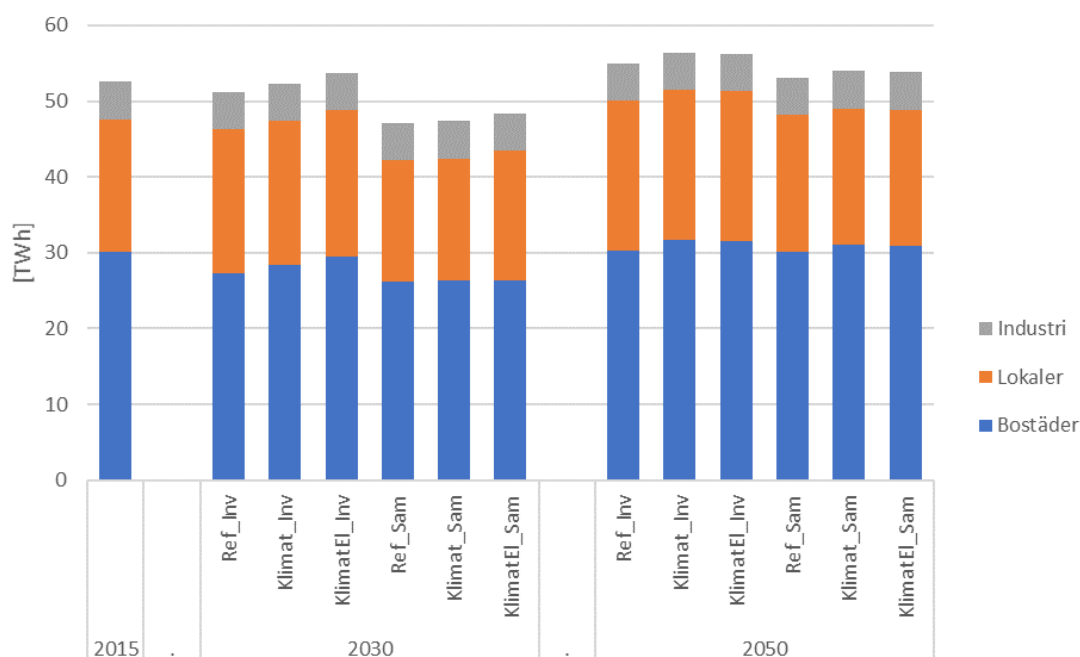
Figur 33. Fjärrvärmeanvändningens utveckling per sektor i grundscenarierna.
