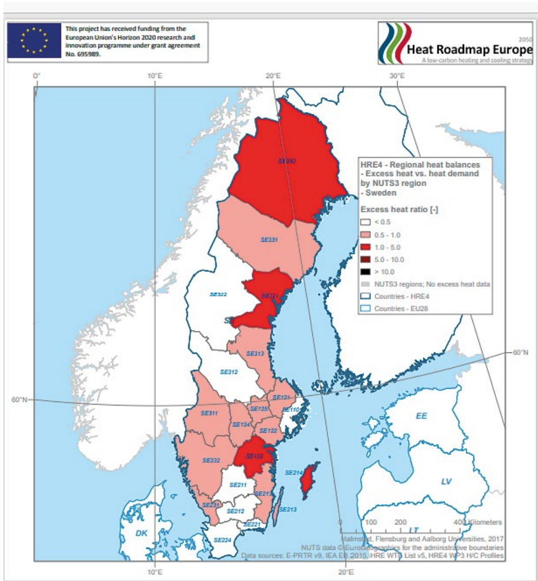
Figur 15. Överskottsvärme (excess heat) vs värmefterfrågan.
