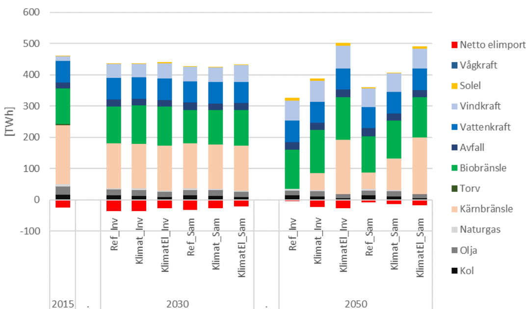
Figur 21. Energitillförsel (primärenergi) till Sverige för grundscenarier.
