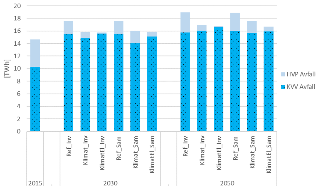
Figur 36. Fjärrvärme från avfallsförbränning fördelat på hetvattenpanna (HVP) och kraftvärme (KVV).
