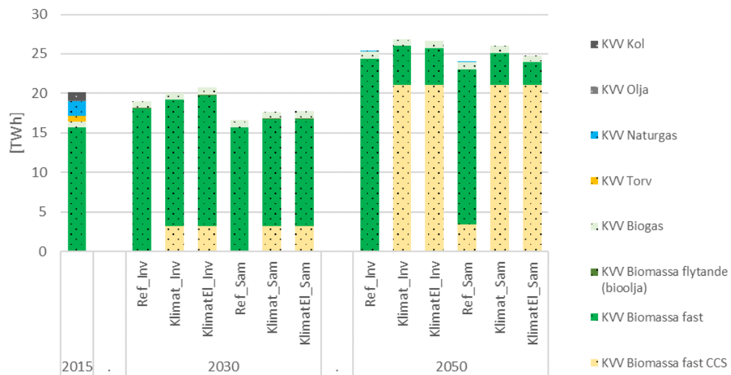
Figur 35. Fjärrvärme producerad från kraftvärme (exkl. avfall).
