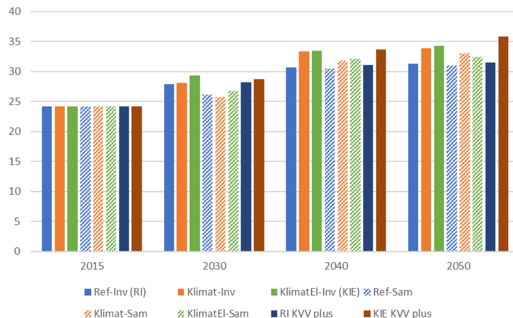
Figur 43. Primärenergibesparingar från grundscenarier och scenarier med mer kraftvärme, EU-beräkningsmetod.
