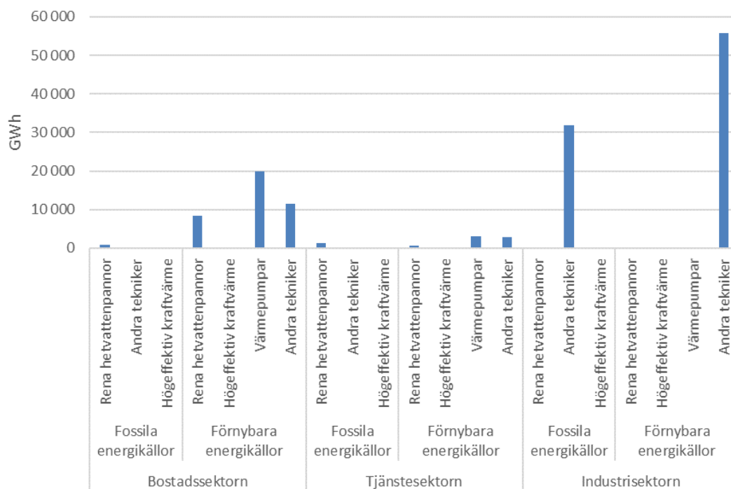
Figur 2. Internt tillhandahållen värme, GWh/år, 2018.
