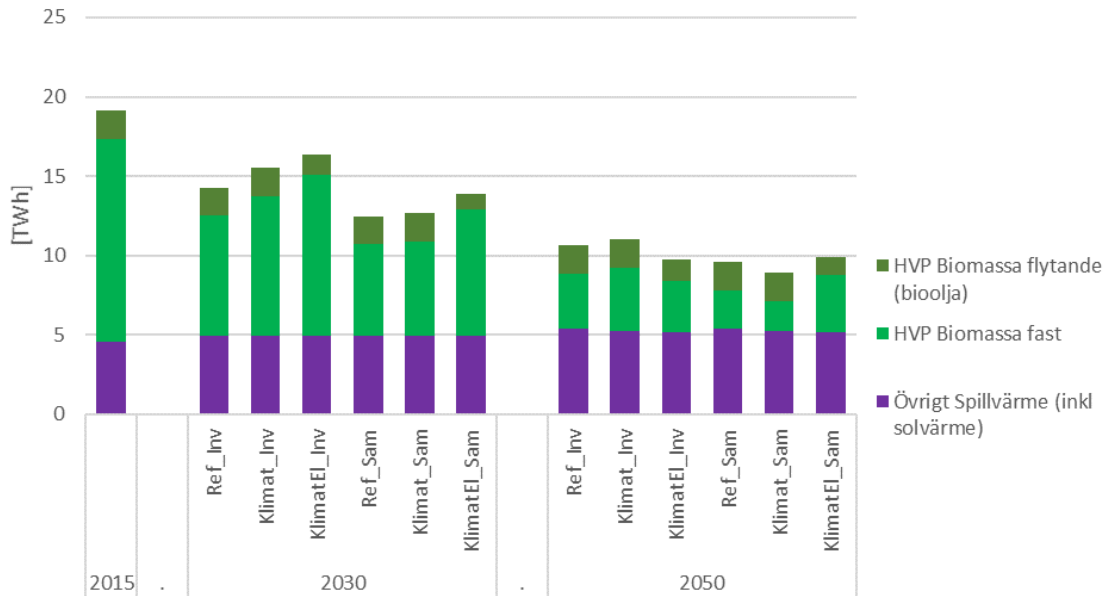
Figur 38. Förnybar fjärrvärme från hetvattenpanna (HVP) samt industriell spillvärme.
