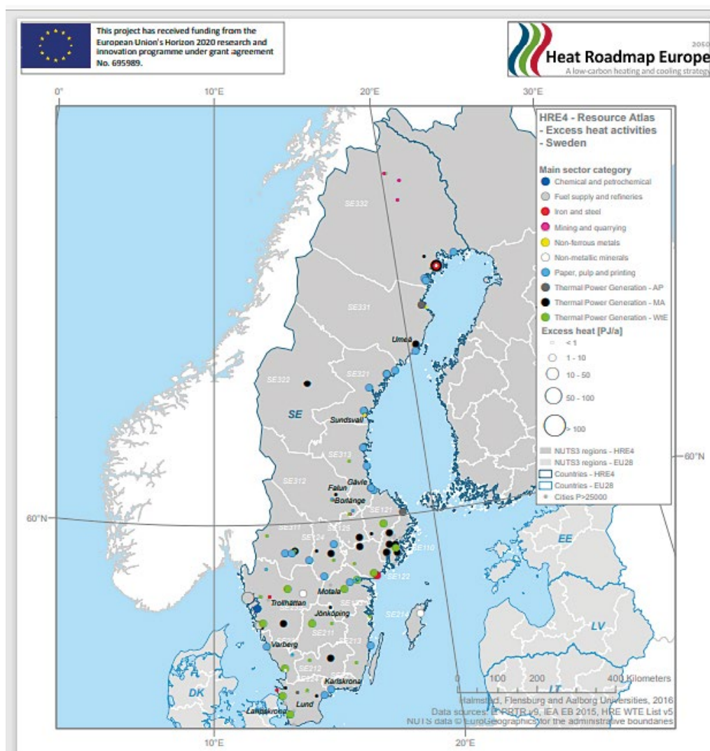
Figur 13. Potentiella källor för spillvärmeanvändning.
