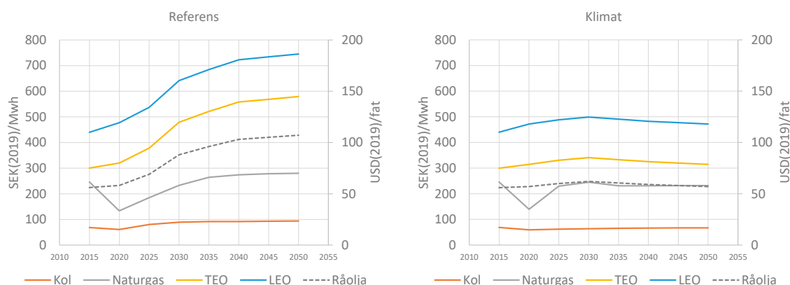
Figur 51. Fossila bränslepriser (SEK 2016 /MWh, fritt nationsgräns och exklusive skatt).
