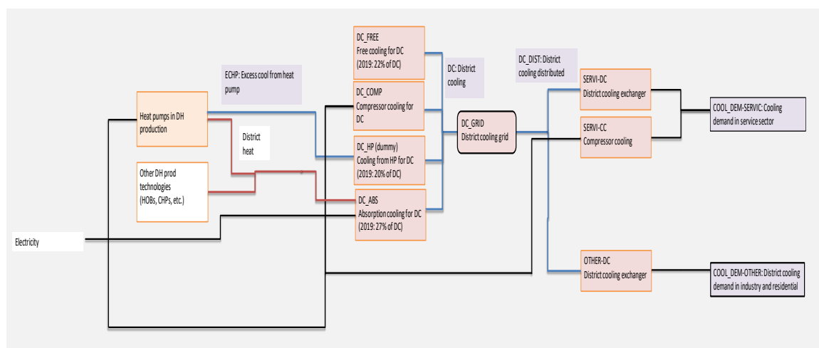
Figur 57. Schematisk bild av modellrepresentationen av kyla.
