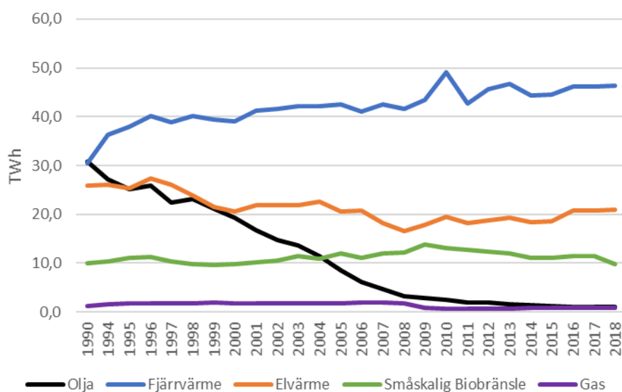
Figur 4. Total energianvändning för uppvärmning och varmvatten 1990–2018, fördelat på använt energislåg, TWh.
