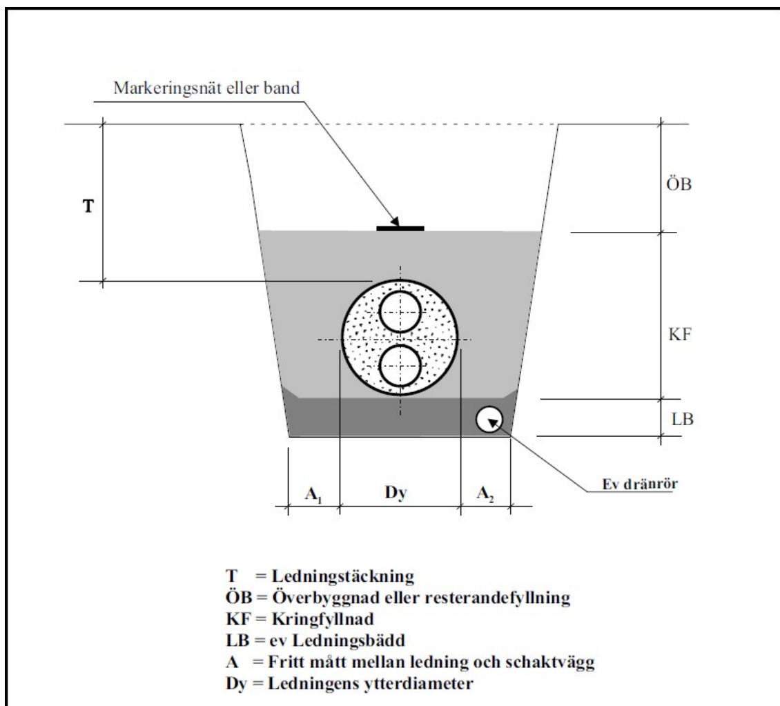
Bild 4. Tvillingrör
