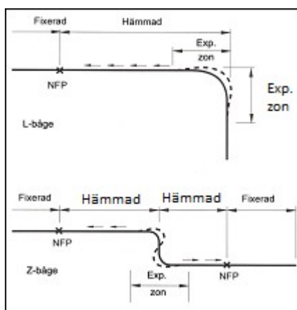
Bild 10. Expansionszon
