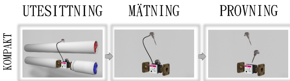
Figur 6. Kompaktmätare
