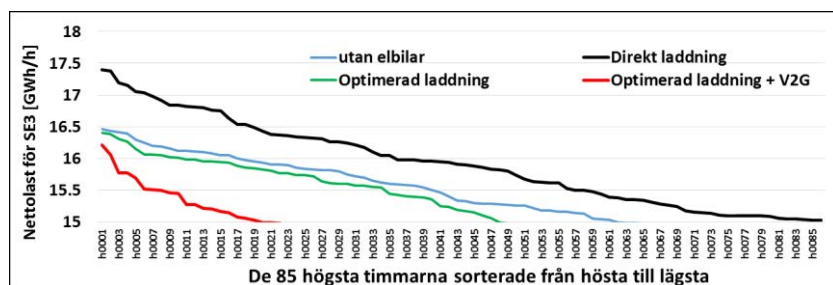
Figur 8.2 Nettolastkurvan för elområde SE3 år 2030 för de 85 mest effekbelastade timmarna under året
