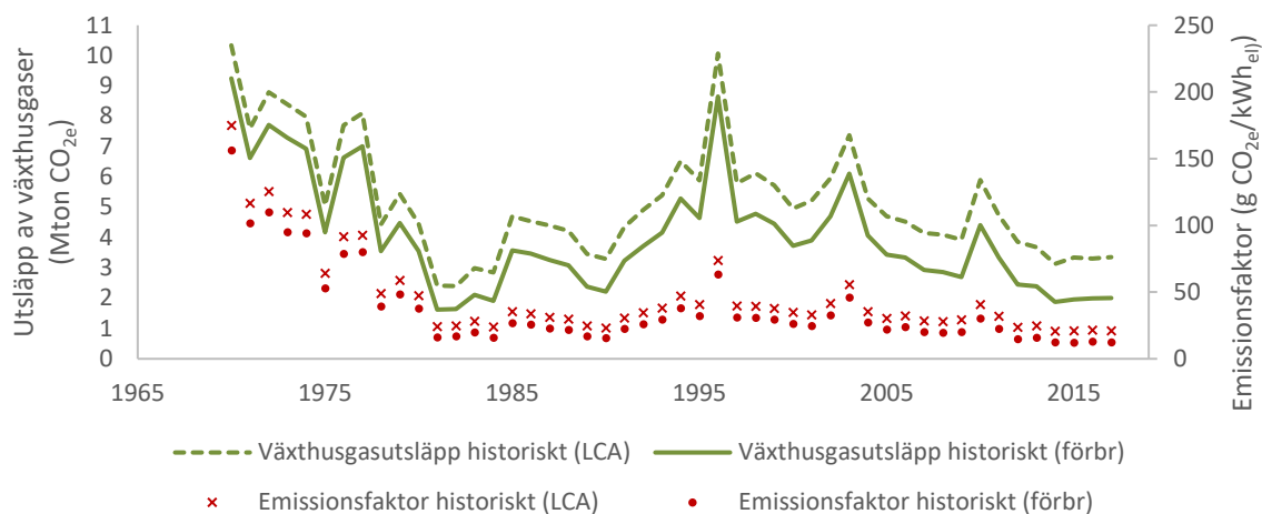
Figur 34. Historisk klimatpåverkan från svensk elproduktion mätt som utsläpp av växthusgaser (Mton CO 2e ) samt emissionsfaktor (g CO 2e /kWh el ). Värderna visas både för enbart direkta utsläpp vid förbränning och som utsläpp i livscykelperspektiv.
