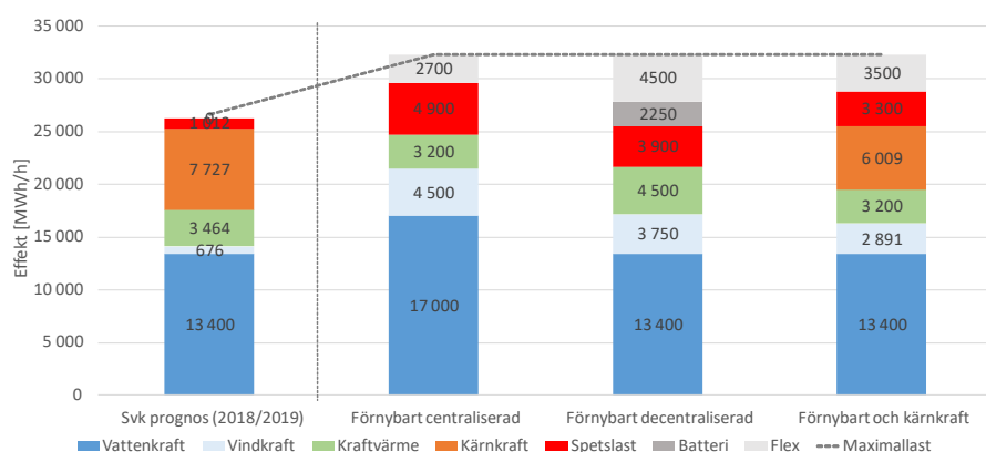
Figur 11: Tillgänglig effekt och topplast enligt Svks metodologi
