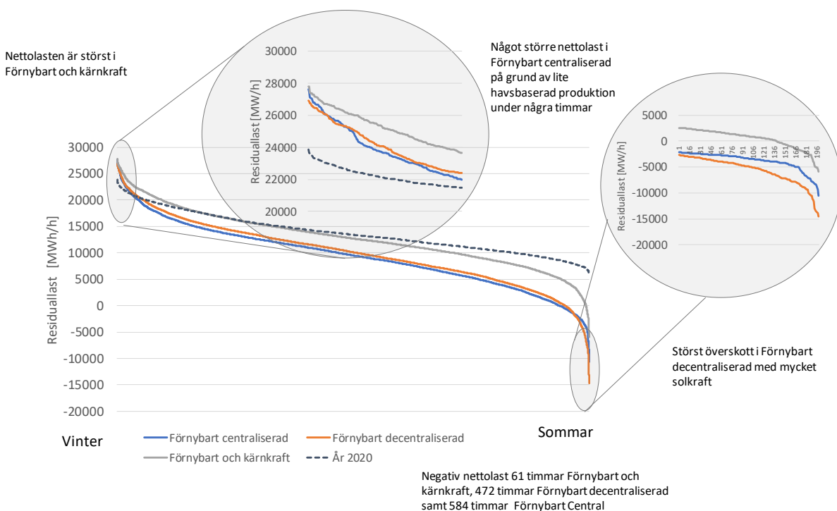
Figur 52: Nettolasten för de tre scenarierna år 2045
